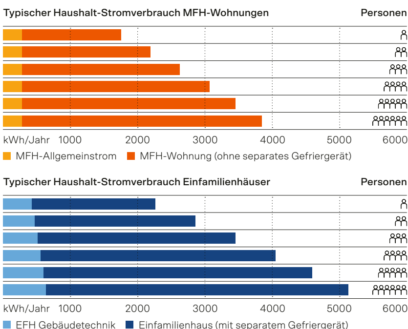
Grafik 1: Stromverbrauch nach Wohnobjekt
